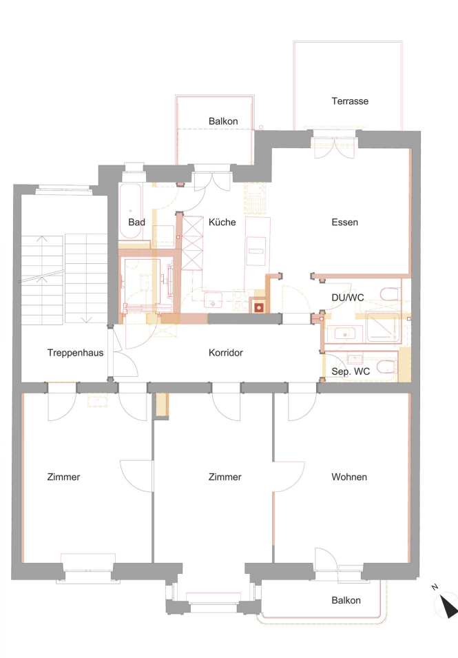
Grundriss 1. Obergeschoss
