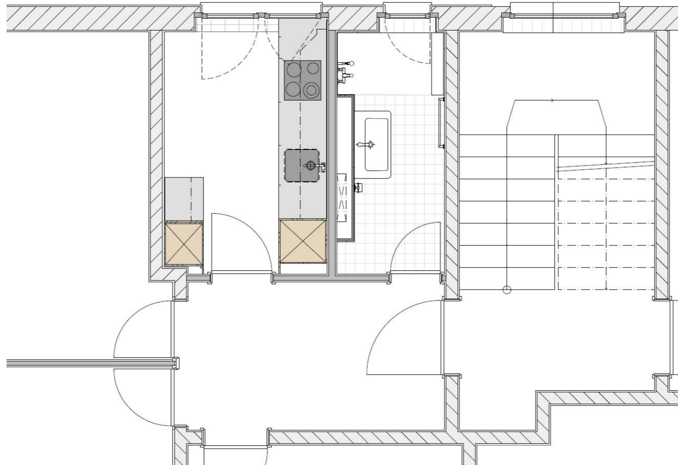
Grundriss Küche, Bad
