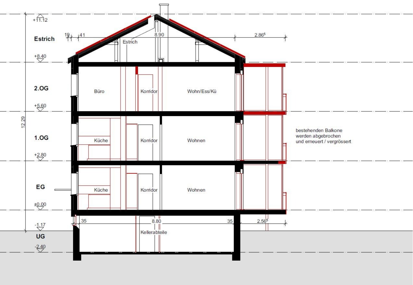
Querschnitt
