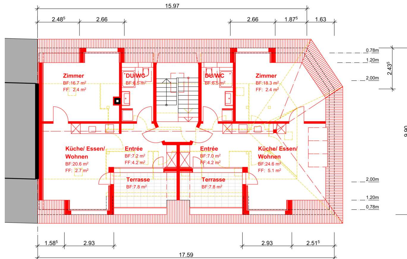
Grundriss
